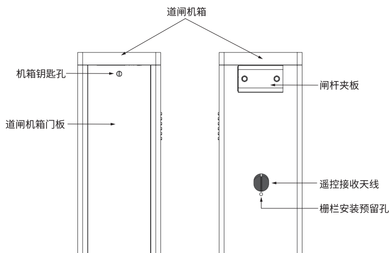
图1-2 外部结构图
