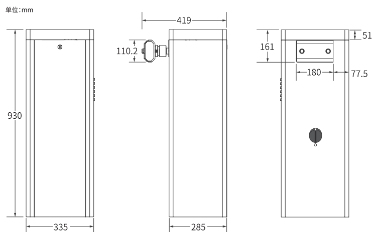
图1-1 产品尺寸图
