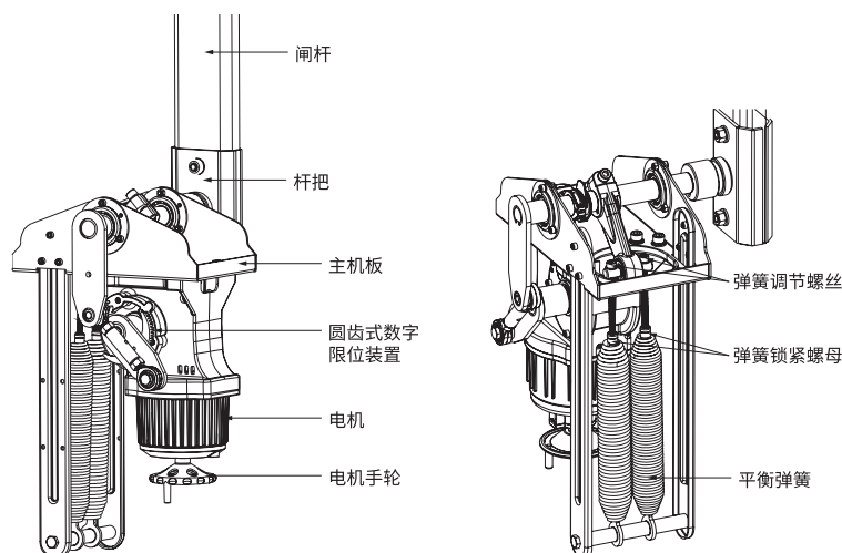
图1-3 道闸机芯展示图
